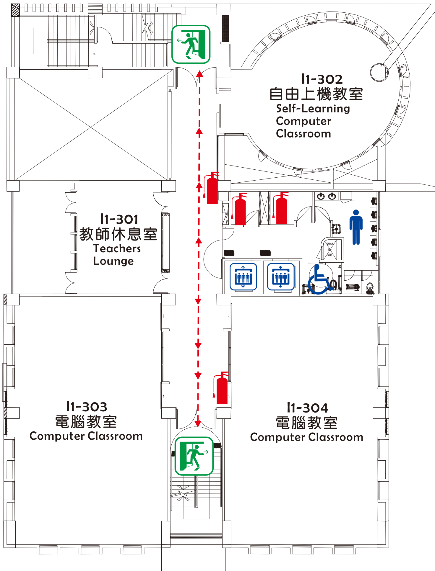
三樓平面圖
